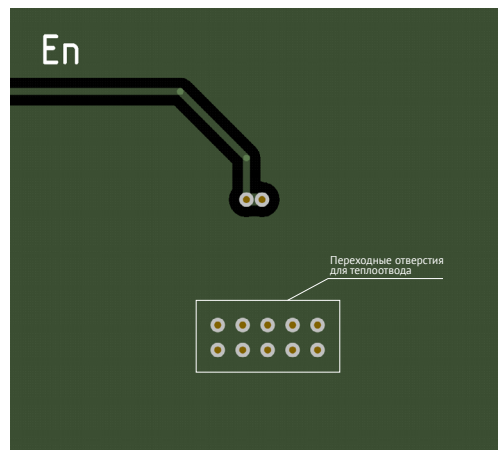
Рис. 23. «Bottom» печатной платы (пример, фрагмент платы).
