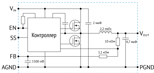
Рис. 2. Упрощённая структурная схема VNA3L0,870SQ.
