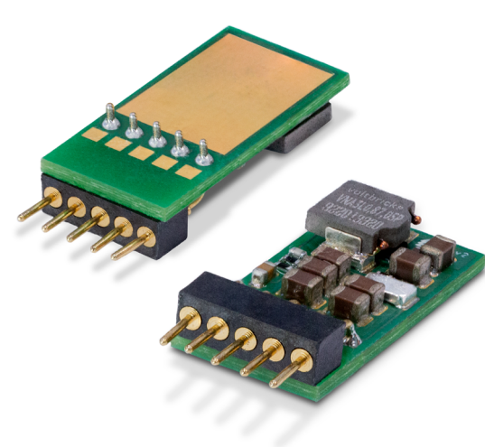
Рис. 29. Внешний вид VNA3L0, 87,0SP.
