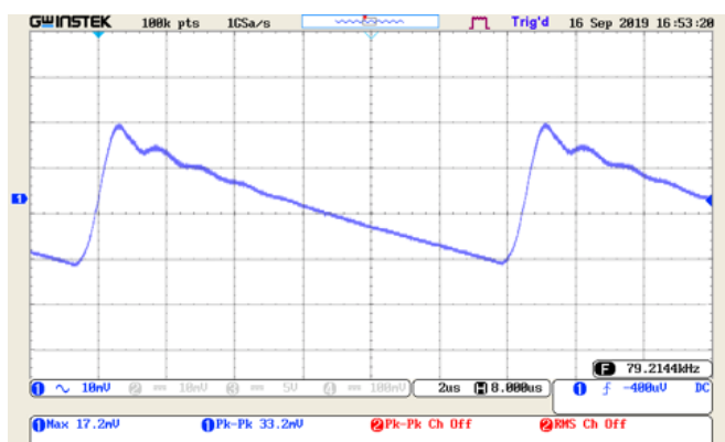
Рис. 9. I_{OUT} = 0,1 A.
