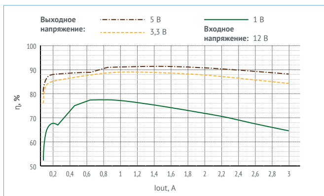
Рис. 12. V_{IN} = 12 В; V_{OUT} = 1 В; 3,3 В; 5 В.
