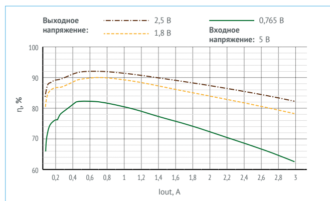
Рис. 13. V_{IN} = 5 В; V_{OUT} = 0,765 В; 1,8 В; 2,5 В.
