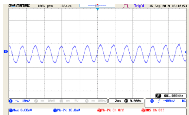
Рис. 10. I_{OUT} = 3 A.
