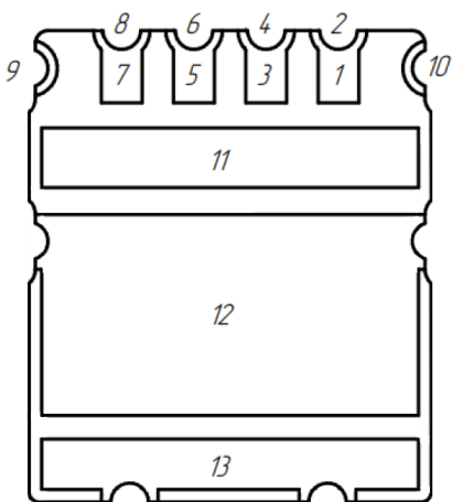
Рис. 1. Расположение выводов модуля VNA3L0,870SQ (вид снизу).
