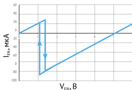
Рис. 16. Типовой гистерезис включения/выключения модуля по выводу EN.
