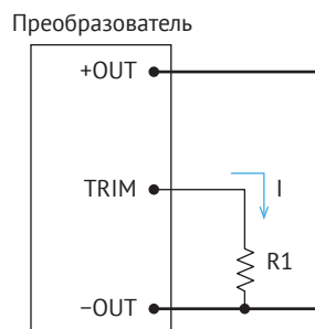
Рис. 7. Регулировка увеличением U_{вых} .
