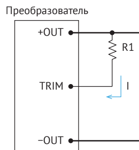
Рис. 8. Регулировка снижением U_{вых} .
