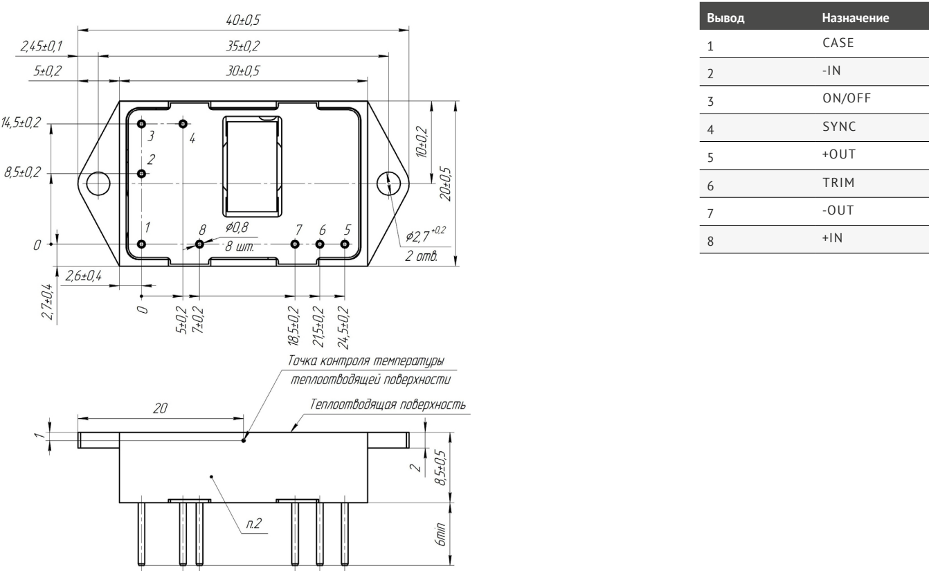
Рис. 10. Одноканальное исполнение с фланцами.
