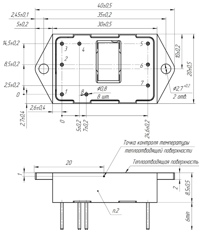
Рис. 11. Двухканальное исполнение с фланцами.
