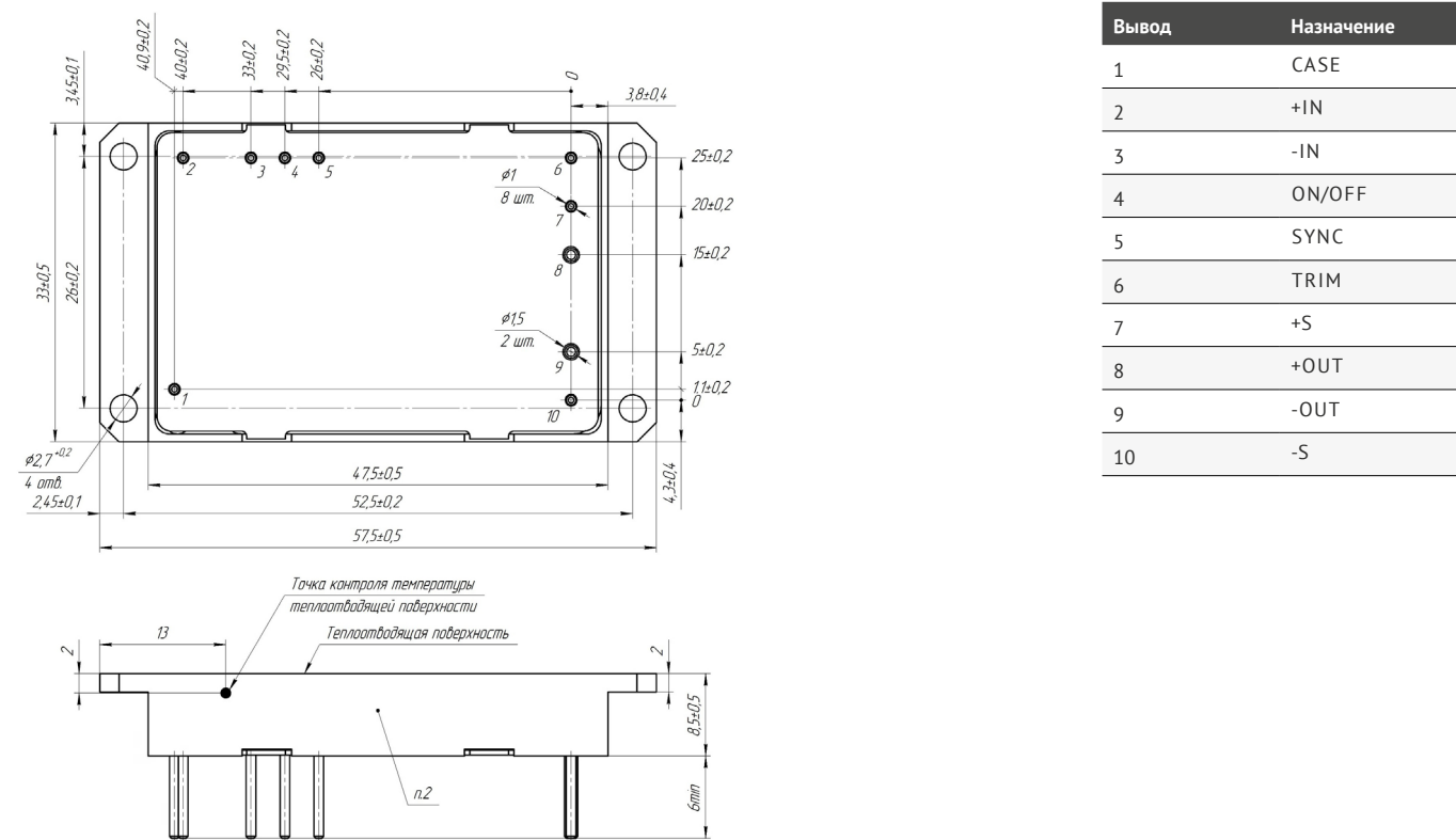
Рис. 12. Одноканальное исполнение.
