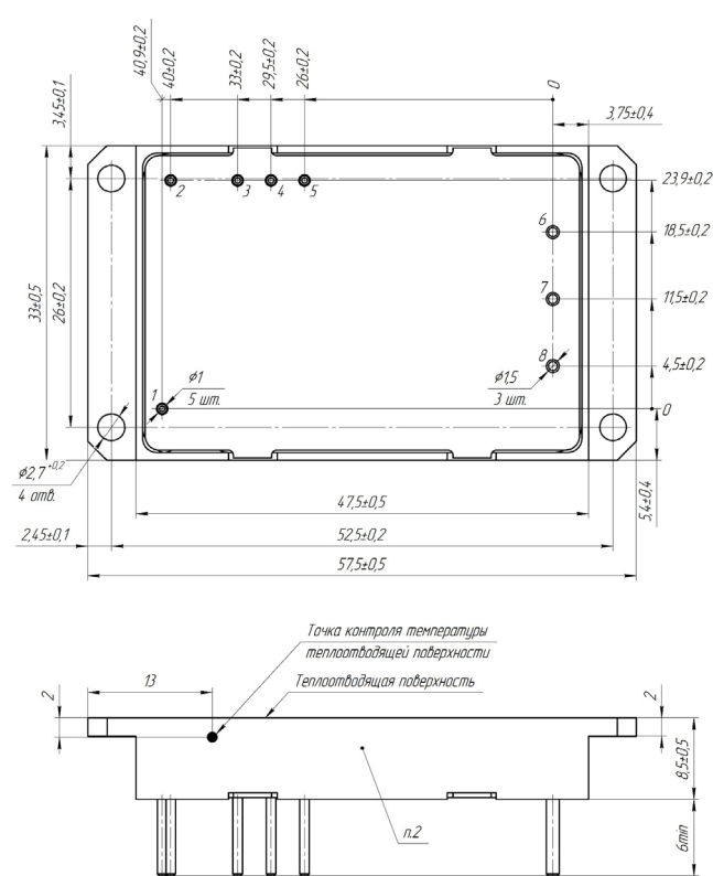
Рис. 13. Двухканальное исполнение.
