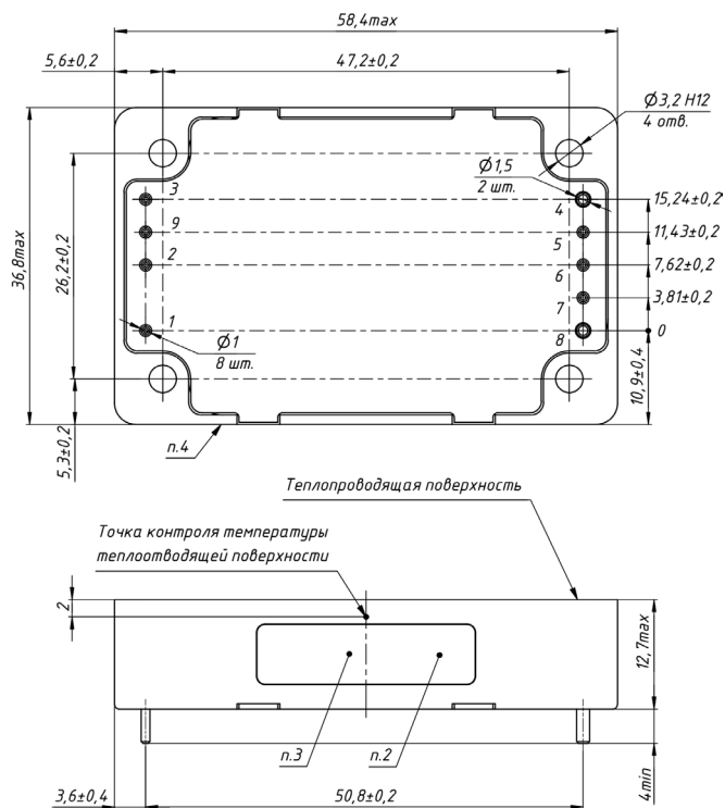
Рис. 2. Исполнение VDMC200.
