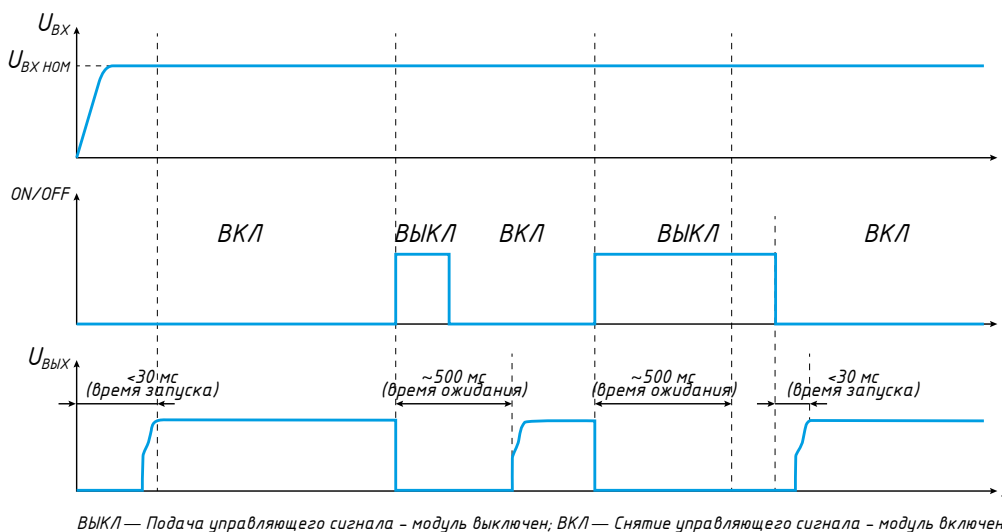
Рис. 8. Циклограмма режима работы дистанционного выключения модулей VDMC25.
