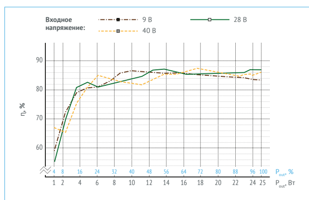
Рис. 12. VDMC25B05.
