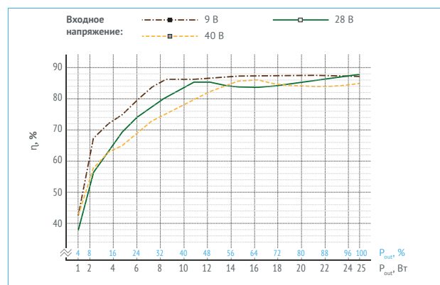
Рис. 17. VDMC25B48.
