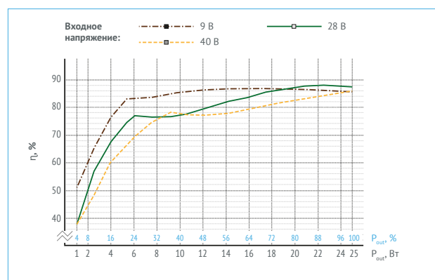
Рис. 16. VDMC25B28.
