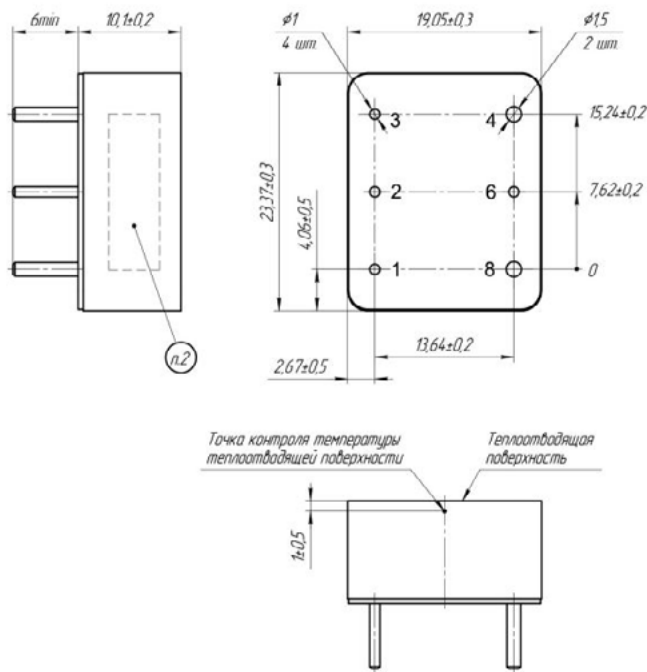
Рис. 18. Исполнение VDMC25.
