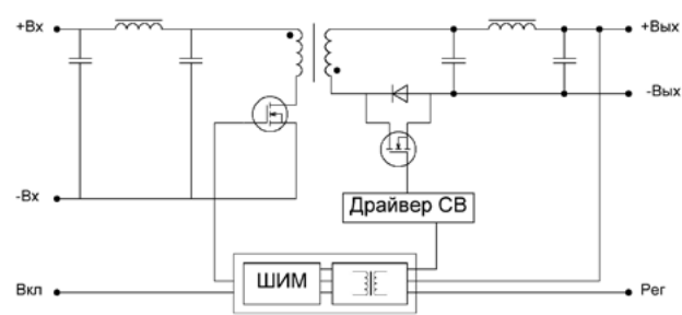
Рис. 1. Функциональная схема VDMC25.
