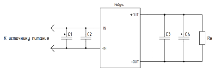
Рис. 2. Типовая схема включения VDMC25.
