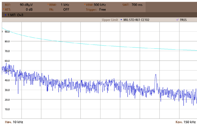
Рис. 22. Спектрограмма соответствия MIL-STD-461 (10–150 kHz).
