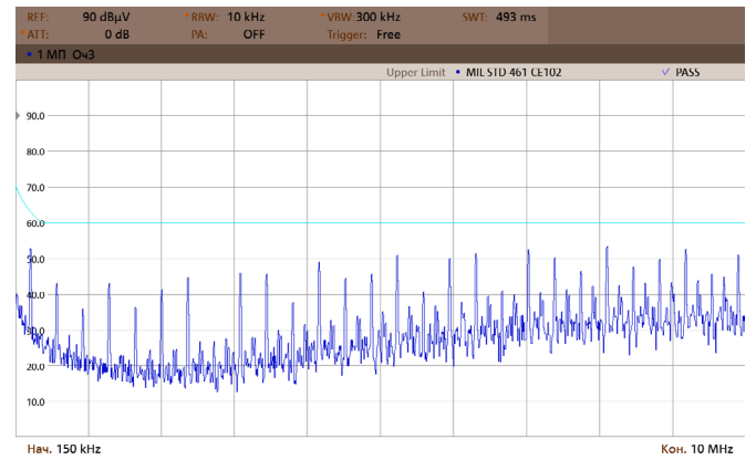
Рис. 23. Спектрограмма соответствия MIL-STD-461 (0,15-10 MHz).
