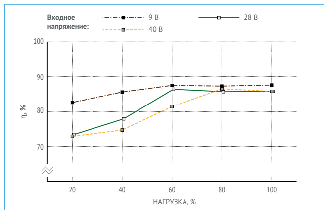
Рис. 16. VDMC50B48.
