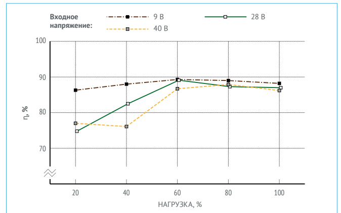
Рис. 13. VDMC50B15.
