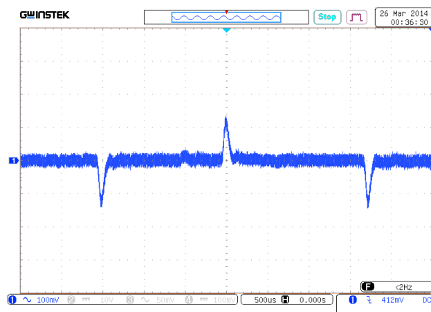
Рис. 21. Переходное отклонение выходного напряжения при изменении выходного тока от 75 до 100%.
