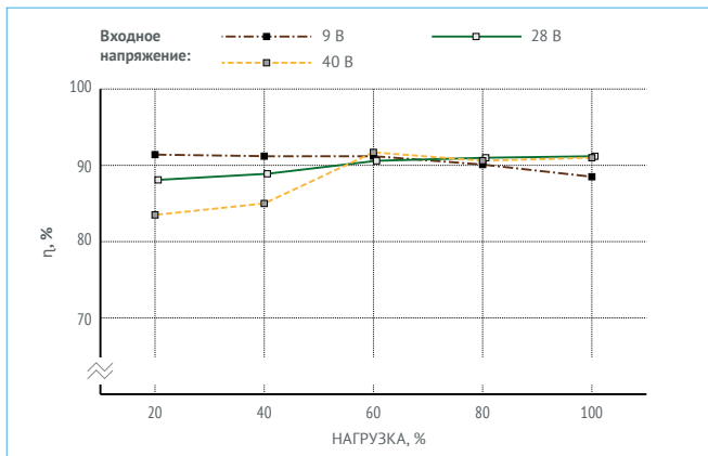
Рис. 10. VDMC50B05.
