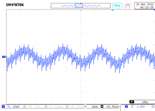
Рис. 20. Пульсации U_{\text{вых.ном}} .
