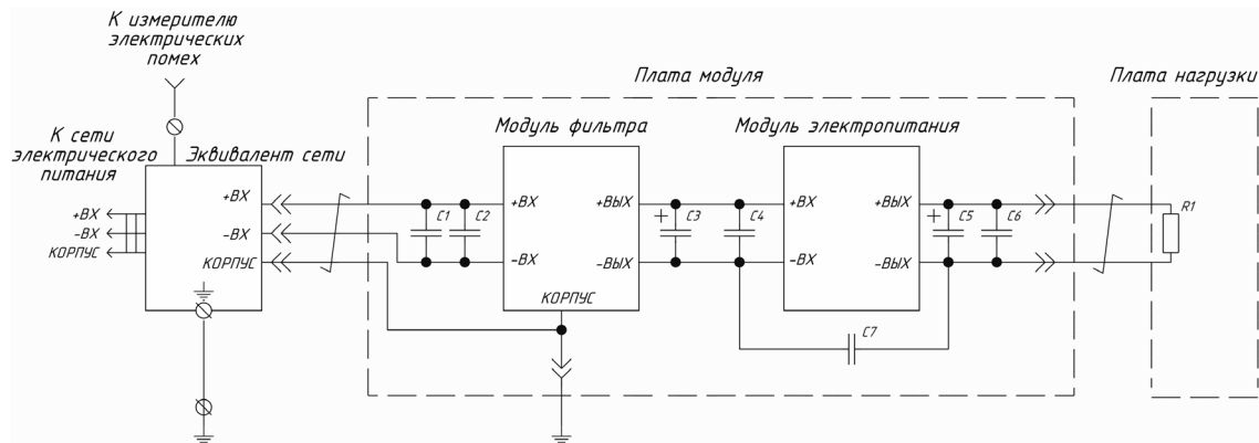
Рис. 3. Схема измерения ЭМС VDMC50.
