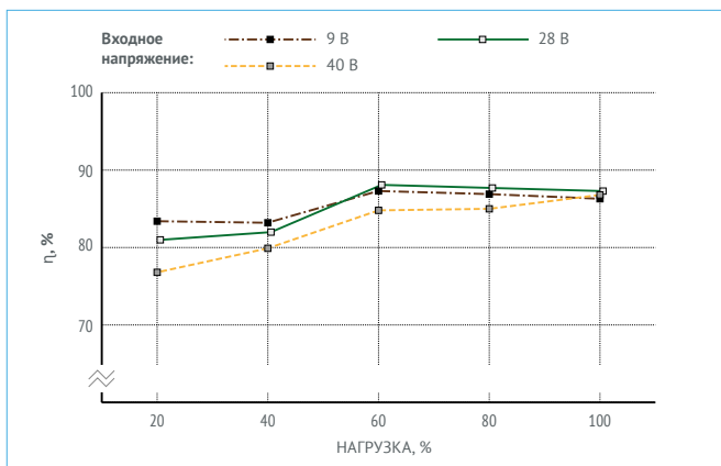
Рис. 14. VDMC50B24.
