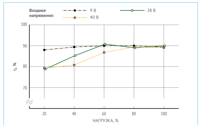
Рис. 12. VDMC50B12.
