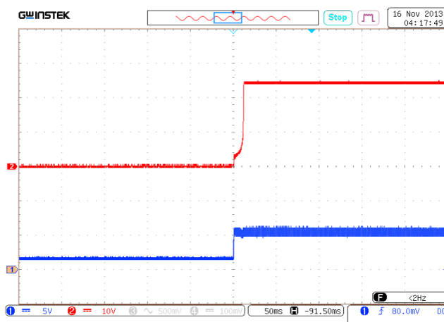
Рис. 18. Установление U_{\text{ВЫХ.НОМ}} с момента подачи ДУ (управляющий сигнал).
