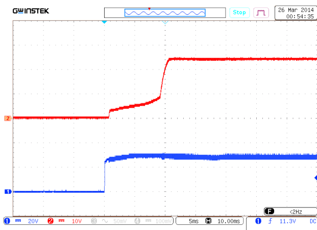
Рис. 19. Установление U_{\text{вых.ном}} с момента подачи U_{\text{вх.ном}} .
