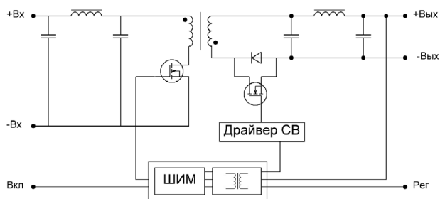
Рис. 1. Топология VDMC50.
