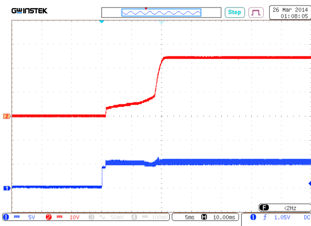
Рис. 17. Установление U_{\text{ВЫХ.НОМ}} с момента подачи ДУ (соединение выводов «ВКЛ» и «-ВХ»).
