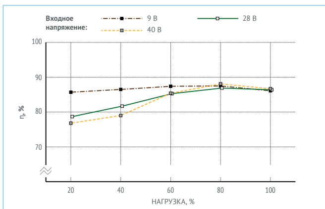
Рис. 15. VDMC50B28.
