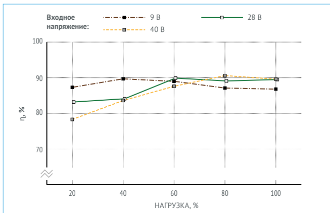
Рис. 11. VDMC50B09.
