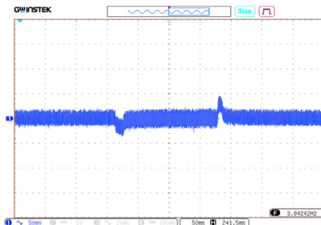
Рис. 7 (г). Осциллограмма переходного отклонения выходного напряжения при изменении выходного тока.
