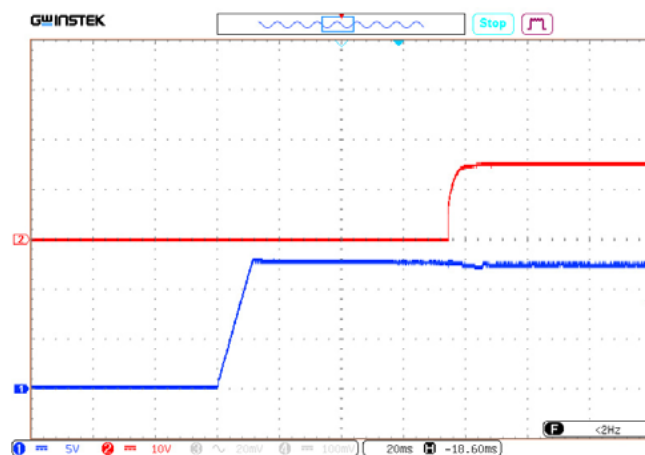
Рис. 7 (б). Осциллограмма установления выходного напряжения с момента подачи входного напряжения.
