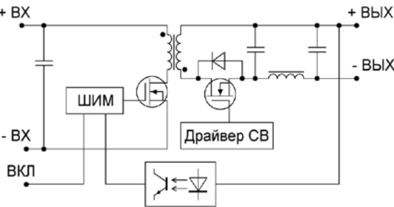
Рис. 1. Топология VDN10.
