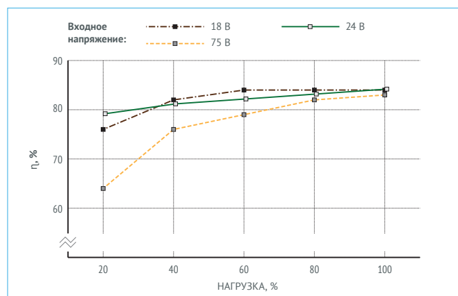
Рис. 5 (г). КПД VDN10W12.
