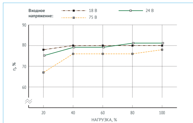
Рис. 5 (б). КПД VDN10W05.
