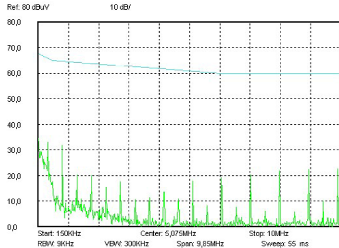
Рис. 9 (а). Спектрограмма 0,15–10 МГц.
