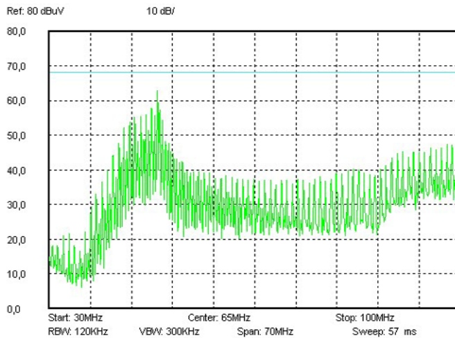
Рис. 9 (в). Спектрограмма 30–100 MHz.
