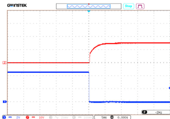
Рис. 7 (а). Осциллограмма установления выходного напряжения с момента подачи команды дистанционного управления.
