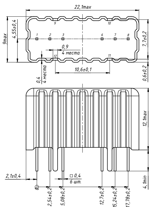
Рис. 11. Стандартное исполнение VDN10.
