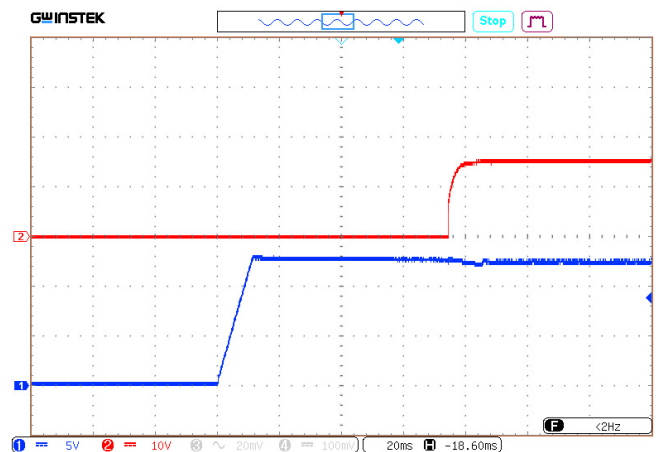
Рис. 8 (б). Осциллограмма установления выходного напряжения с момента подачи входного напряжения.
