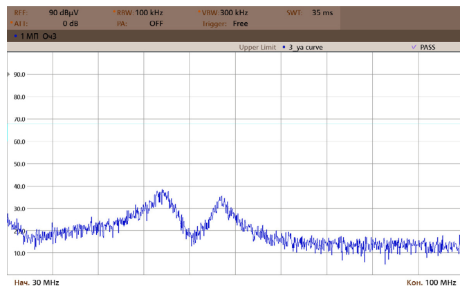
Рис. 40. Диапазон 30..100 МГц.
