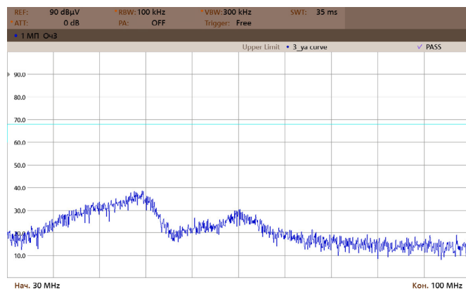
Рис. 36. Диапазон 30..100 МГц.
