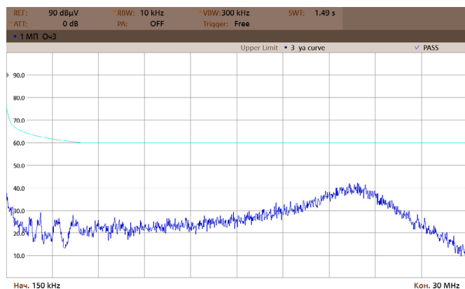
Рис. 35. Диапазон 0,15..30 МГц.
