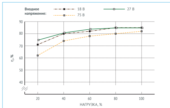
Рис. 6 (д). КПД VDR50W24.
