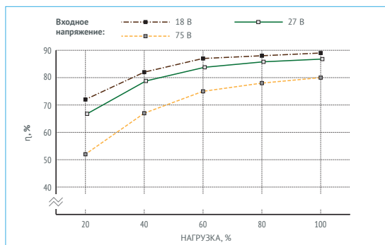
Рис. 6 (а). КПД VDR50W05.
