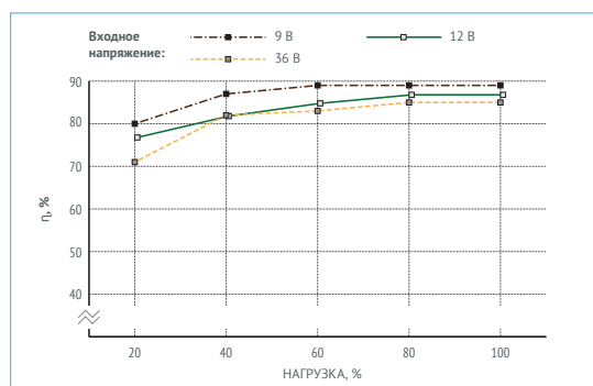
Рис. 7 (г). КПД VDR50B24.
