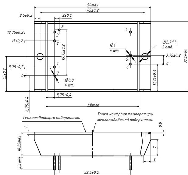
Рис. 13. Исполнение в усиленном корпусе с фланцами.
