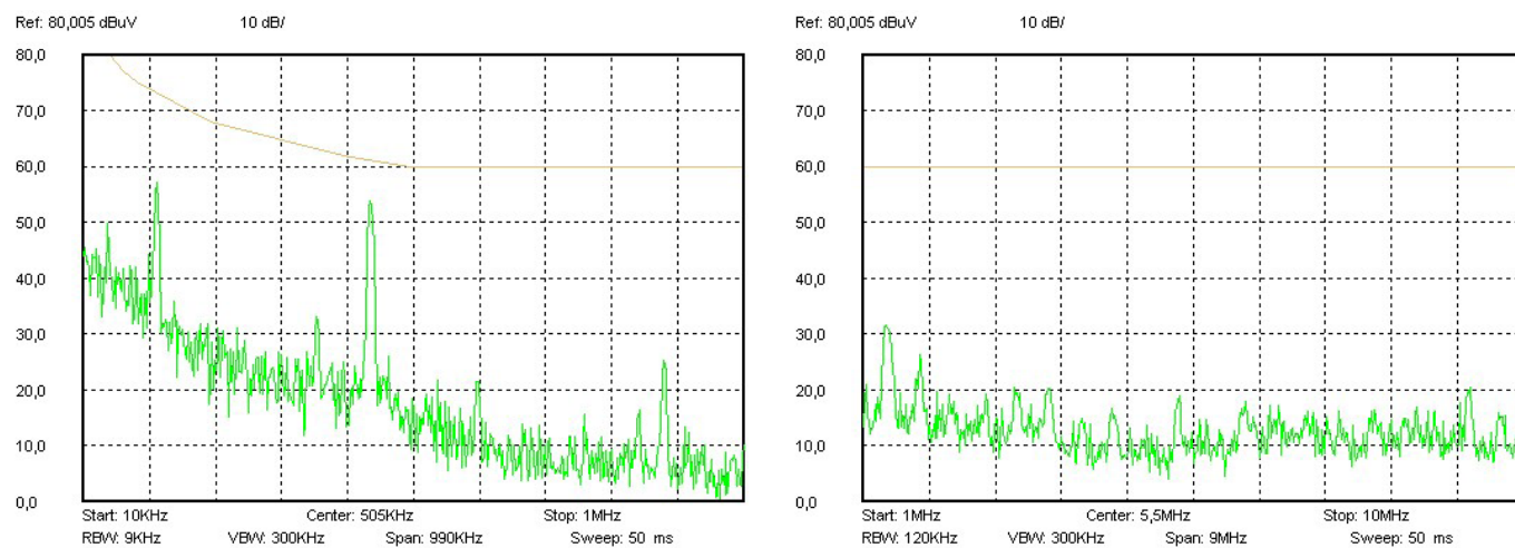
Рис. 11 (а). Спектрограммы 0,01–10 MHz.
