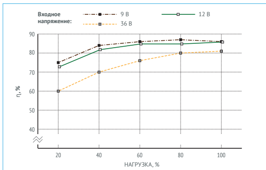
Рис. 7 (д). КПД VDR50B28.
