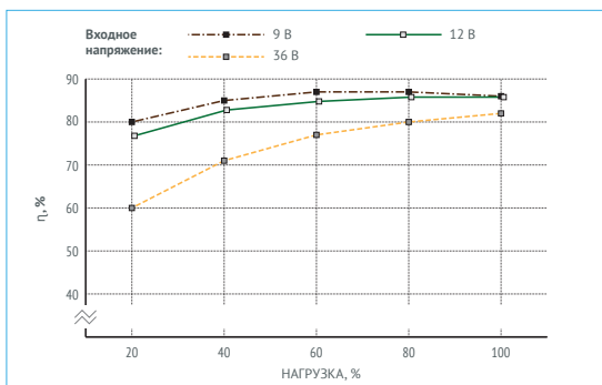
Рис. 7 (а). КПД VDR50B3.3.
