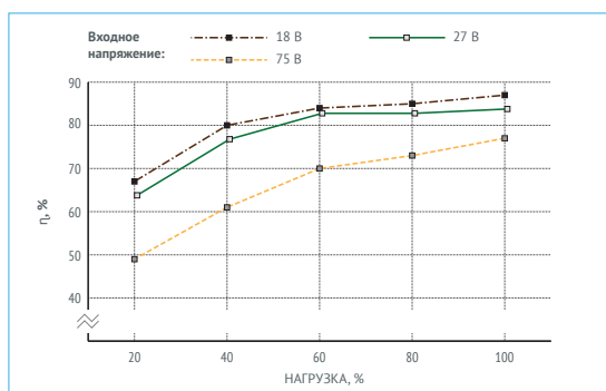
Рис. 6 (в). КПД VDR50W12.
