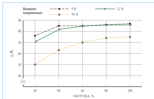
Рис. 7 (б). КПД VDR50B12.
