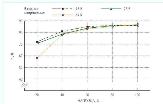
Рис. 6 (е). КПД VDR50W28.
