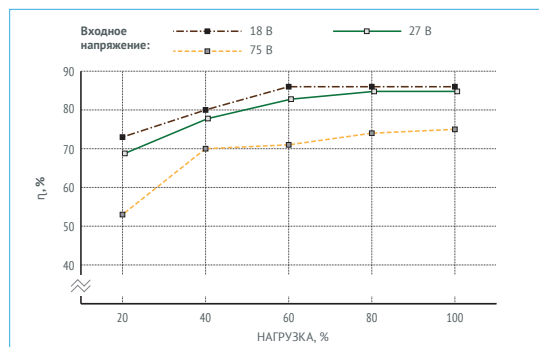
Рис. 6 (б). КПД VDR50W09.
