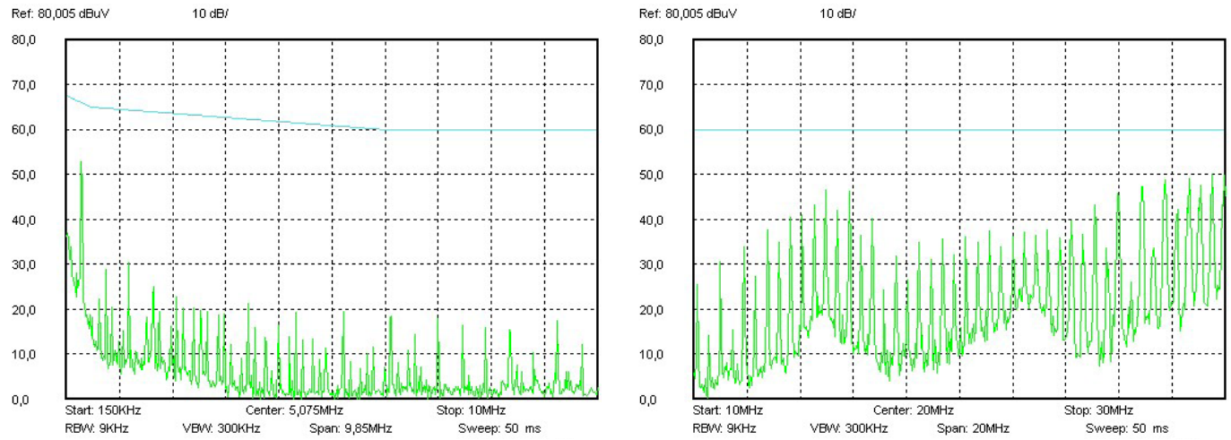
Рис. 10 (а). Спектрограммы 0,01–10 MHz.
