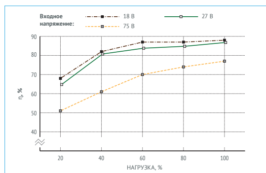
Рис. 6 (г). КПД VDR50W15.
