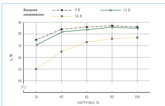
Рис. 7 (в). КПД VDR50B15.
