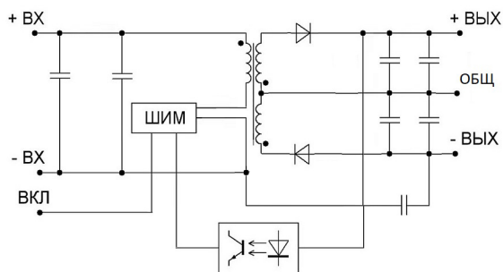
Рис. 2. Функциональная схема для двухканального исполнения VDR11.
