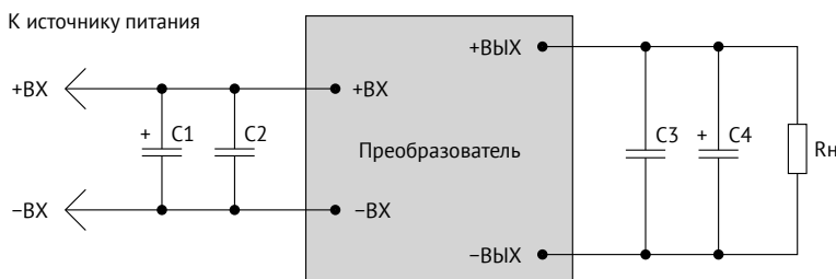
Рис. 3. Типовая схема включения VDR11 для одноканального исполнения.
