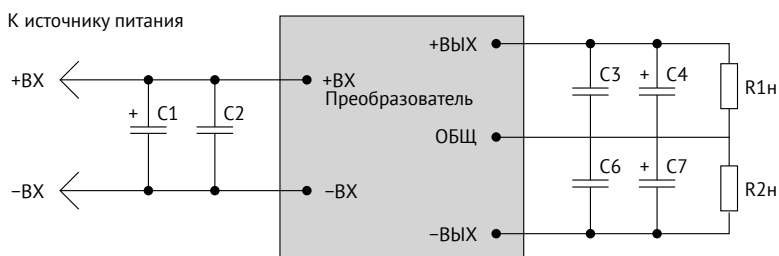
Рис. 4. Типовая схема включения VDR11 для двухканального исполнения.
