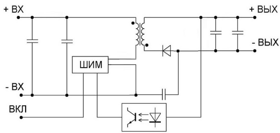
Рис. 1. Функциональная схема для одноканального исполнения VDR11.
