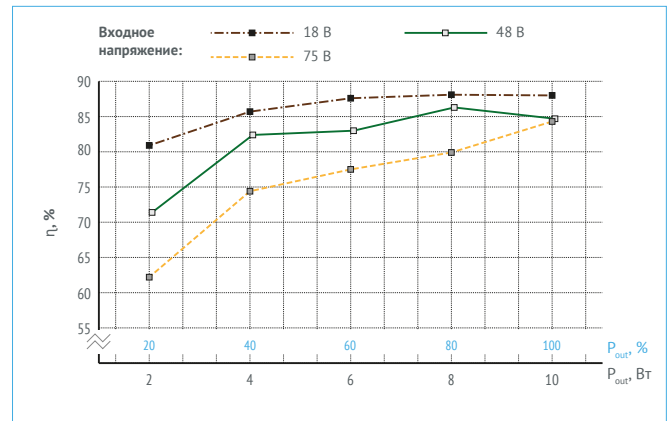
Рис. 30. КПД для VDRI10W24.
