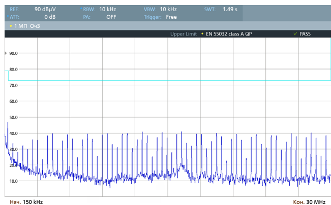
Рис. 69. Спектрограмма работы VDRI10B12 по схеме включения [Рис. 3], измерения произведены в соответствии с EN 55032 Class A (0,15–30 МГц).
