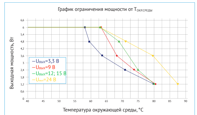
Рис. 32. График ограничения мощности от T_{окр.среды} без применения внешнего радиатора. Для модулей VDRI6W с входной сетью «W», при U_{BX}=48 В .
