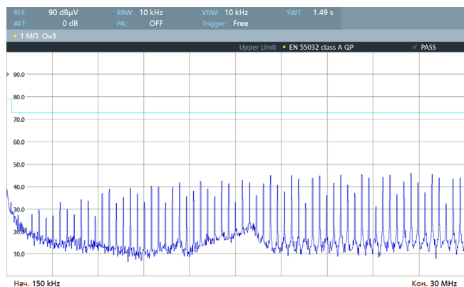
Рис. 71. Спектрограмма работы VDRI10B24 по схеме включения [Рис. 3], измерения произведены в соответствии с EN 55032 Class A (0,15–30 МГц).
