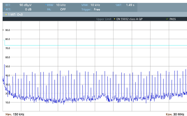
Рис. 65. Спектрограмма работы VDRI10B3,3 по схеме включения [Рис. 3], измерения произведены в соответствии с EN 55032 Class A (0,15–30 МГц).
