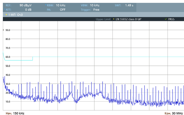
Рис. 46. Спектрограмма работы VDRI6B05 по схеме включения [Рис. 4], измерения произведены в соответствии с EN 55032 Class B (0,15–30 МГц).
