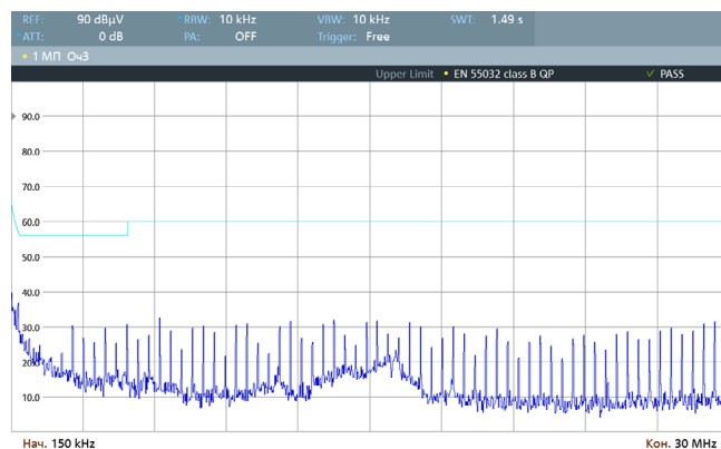
Рис. 68. Спектрограмма работы VDRI10B05 по схеме включения [Рис. 4], измерения произведены в соответствии с EN 55032 Class B (0,15–30 МГц).
