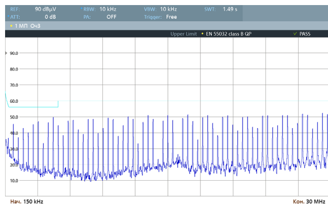
Рис. 72. Спектрограмма работы VDRI10B24 по схеме включения [Рис. 4], измерения произведены в соответствии с EN 55032 Class B (0,15–30 МГц).
