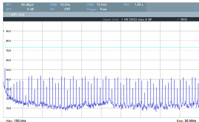
Рис. 43. Спектрограмма работы VDRI6B3,3 по схеме включения [Рис. 3], измерения произведены в соответствии с EN 55032 Class A (0,15–30 МГц).
