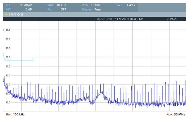
Рис. 70. Спектрограмма работы VDRI10B12 по схеме включения [Рис. 4], измерения произведены в соответствии с EN 55032 Class B (0,15–30 МГц).
