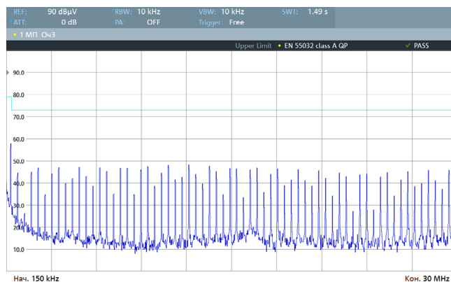
Рис. 75. Спектрограмма работы VDRI10W15 по схеме включения [Рис. 3], измерения произведены в соответствии с EN 55032 Class A (0,15–30 МГц).
