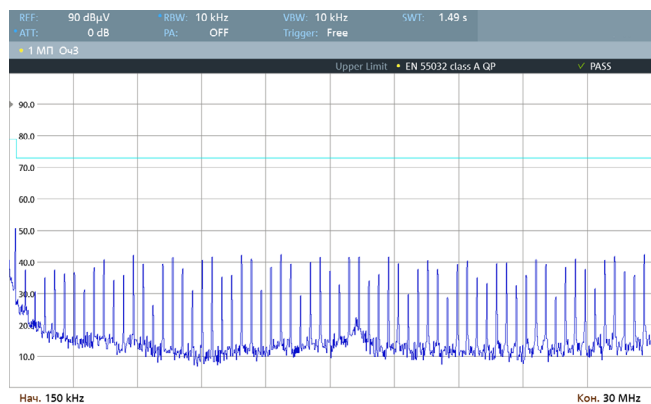
Рис. 45. Спектрограмма работы VDRI6B05 по схеме включения [Рис. 3], измерения произведены в соответствии с EN 55032 Class A (0,15–30 МГц).
