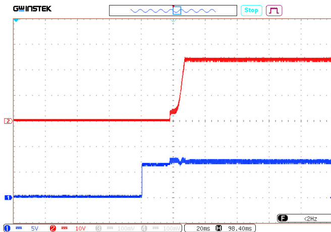
Рис. 39. Установление U_{\text{вых.ном}} с момента подачи сигнала ДУ (размыкание выводов «ДУ» и «-ВХ») Луч 1 (синий) – напряжение на выводе «ДУ». Масштаб 5 В/дел. Луч 2 (красный) – выходное напряжение. Масштаб 10 В/дел. Развертка 20 мс/дел.
