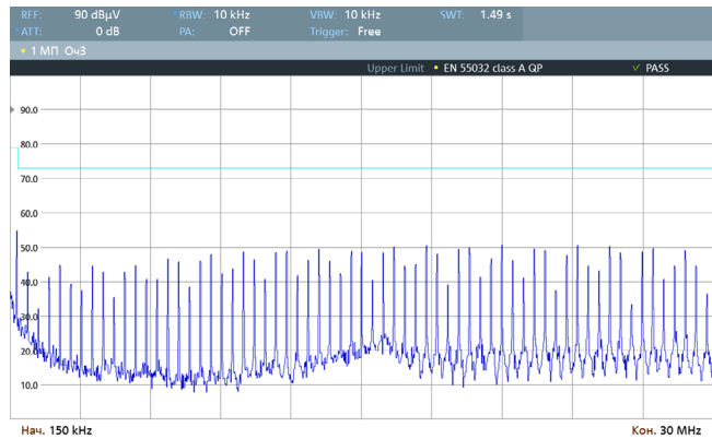
Рис. 77. Спектрограмма работы VDRI10W24 по схеме включения [Рис. 3], измерения произведены в соответствии с EN 55032 Class A (0,15–30 МГц).
