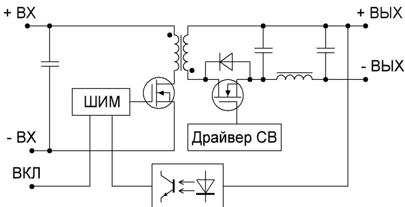
Рис. 1. Функциональная схема VDRI6, VDRI10.
