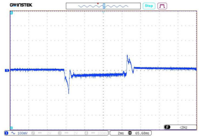
Рис. 36. Осциллограмма переходного отклонения выходного напряжения при скачкообразном изменении выходного тока с 50% до 100% и со 100% до 50%.
