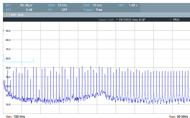
Рис. 64. Спектрограмма работы VDRI6W24 по схеме включения [Рис. 4], измерения произведены в соответствии с EN 55032 Class B (0,15–30 МГц).
