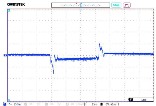
Рис. 40. Осциллограмма переходного отклонения выходного напряжения при скачкообразном изменении выходного тока с 50% до 100% и со 100% до 50%. Масштаб 100 мВ/дел. Развертка 2 мс/дел.
