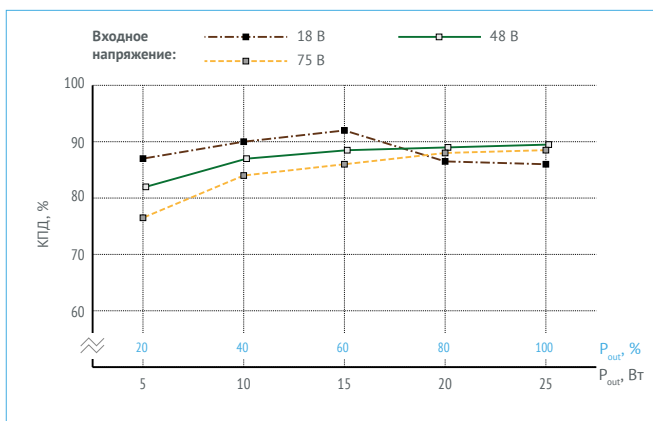
Рис. 33. КПД для VDRI25W09.
