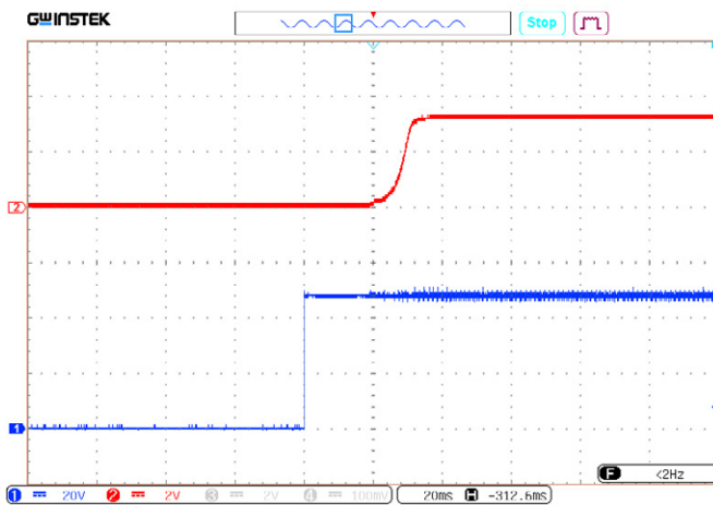
Рис. 54. Установление U_{\text{вых,ном}} с момента подачи U_{\text{вх,ном}} . Луч 1 (синий) – входное напряжение. Масштаб 20 В/дел. Луч 2 (красный) – выходное напряжение. Масштаб 2 В/дел. Развертка 20 мс/дел.
