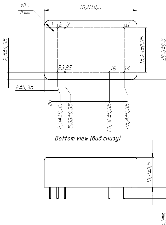
Рис. 64. Исполнение VDRI15, VDRI25.
