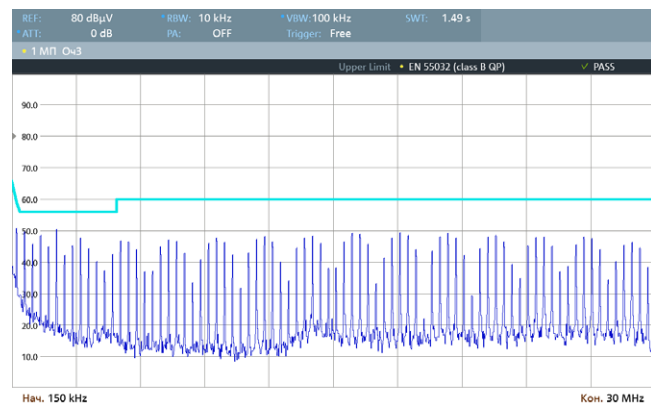
Рис. 59. Спектрограмма работы VDRI15W48 по схеме включения [Рис. 4], измерения произведены в соответствии с EN 55032 Class B (0,15–30 МГц).
