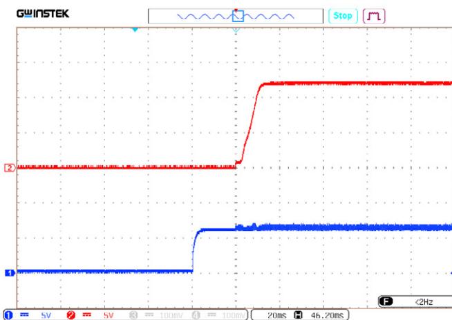
Рис. 48. Установление U_{\text{вых.ном}} с момента подачи сигнала ДУ (соединение выводов «VKЛ» и «-VX»). Луч 1 (синий) – входное напряжение. Масштаб 5 В/дел. Луч 2 (красный) – выходное напряжение. Масштаб 5 В/дел. Развертка 20 мс/дел.
