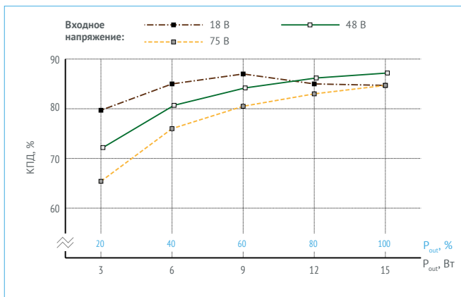
Рис. 20. КПД для VDRI15W09.
