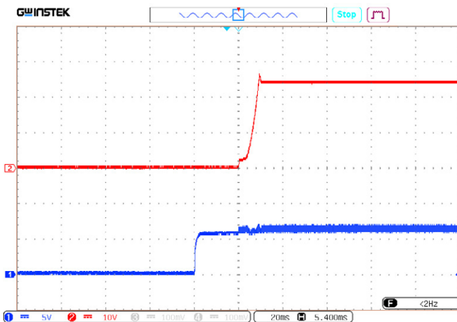
Рис. 44. Установление U_{\text{вых.ном}} с момента подачи сигнала ДУ (соединение выводов «ДУ» и «-VX».) Луч 1 (синий) – входное напряжение. Масштаб 5 В/дел. Луч 2 (красный) – выходное напряжение. Масштаб 10 В/дел. Развертка 20 мс/дел.
