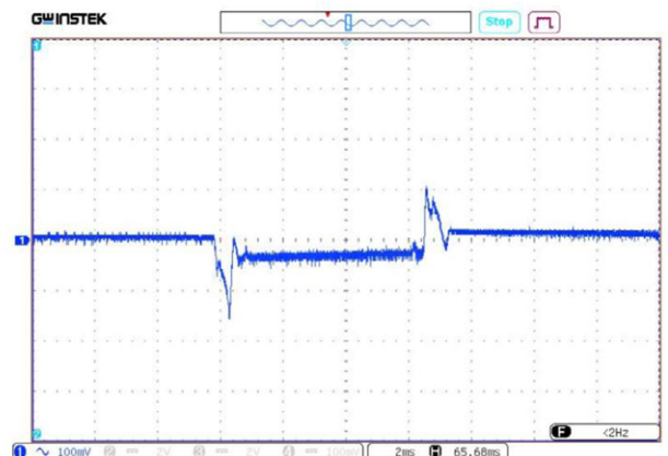
Рис. 53. Осциллограмма переходного отклонения выходного напряжения при скачкообразном изменении выходного тока с 50% до 100% и со 100% до 50%. Масштаб 100 мВ/дел. Развертка 2 мкс/дел.
