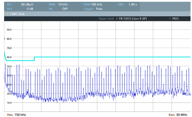
Рис. 63. Спектрограмма работы VDRI25W48 по схеме включения [Рис. 4], измерения произведены в соответствии с EN 55032 Class B (0,15–30 МГц).
