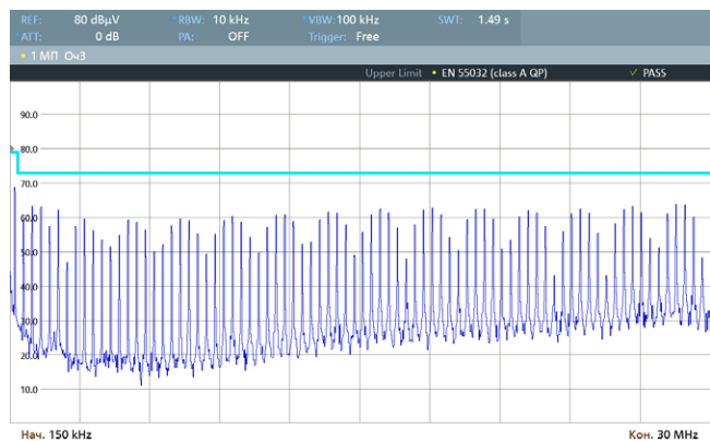
Рис. 58. Спектрограмма работы VDRI15W48 по схеме включения [Рис. 3], измерения произведены в соответствии с EN 55032 Class A (0,15–30 МГц).
