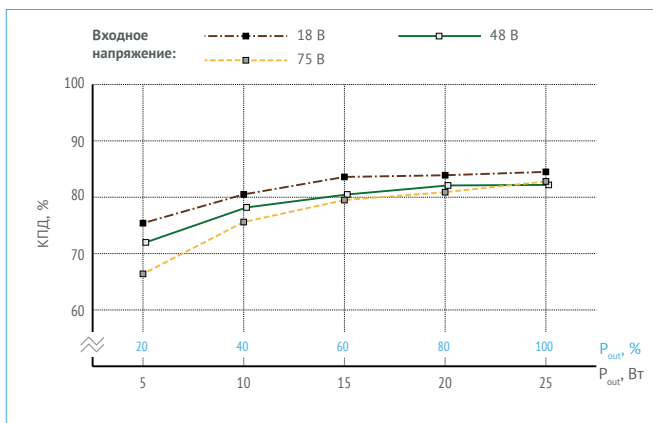
Рис. 31. КПД для VDRI25W3,3.
