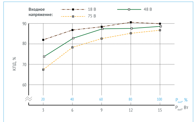
Рис. 21. КПД для VDRI15W12.
