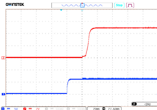
Рис. 40. Установление U_{ВЫХ.НОМ} с момента подачи сигнала ДУ (размыкание выводов «ДУ» и «-ВХ»).
