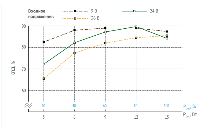
Рис. 15. КПД для VDRI15B15.
