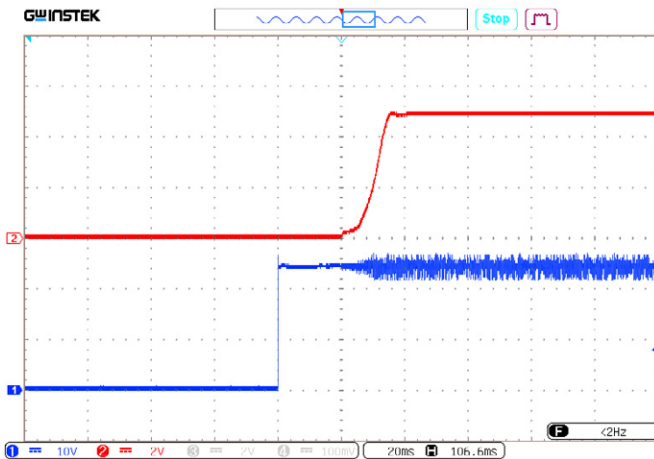
Рис. 42. Установление U_{\text{вых.ном}} с момента подачи U_{\text{вх.ном}} . Луч 1 (синий) – входное напряжение. Масштаб 10 В/дел. Луч 2 (красный) – выходное напряжение. Масштаб 2 В/дел. Развертка 20 мс/дел.
