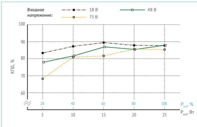
Рис. 36. КПД для VDRI25W24.
