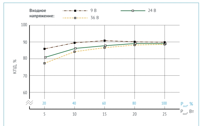
Рис. 27. КПД для VDRI25B12.
