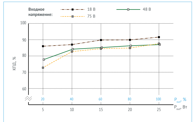
Рис. 37. КПД для VDRI25W48.
