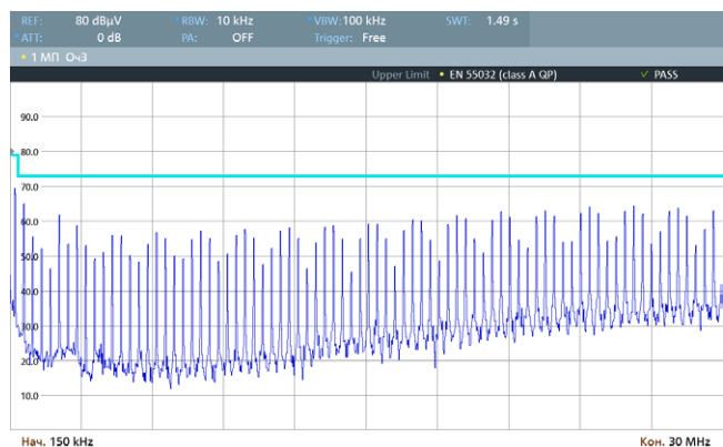
Рис. 60. Спектрограмма работы VDRI25B48 по схеме включения [Рис. 3], измерения произведены в соответствии с EN 55032 Class A (0,15–30 МГц).
