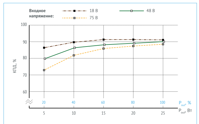
Рис. 34. КПД для VDRI25W12.
