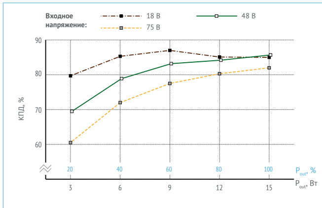
Рис. 19. КПД для VDRI15W05.
