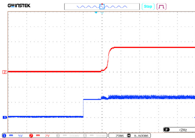
Рис. 52. Установление U_{\text{ВЫХ.НОМ}} с момента подачи сигнала ДУ (соединение выводов «ВКЛ» и «-ВХ» ). Луч 1 (синий) – входное напряжение. Масштаб 5 В/дел. Луч 2 (красный) – выходное напряжение. Масштаб 2 В/дел. Развертка 20 мс/дел.
