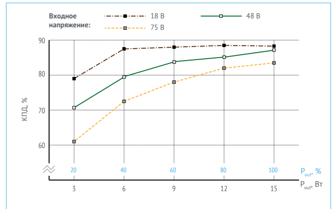
Рис. 22. КПД для VDRI15W15.
