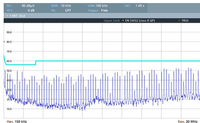
Рис. 61. Спектрограмма работы VDRI25B48 по схеме включения [Рис. 4], измерения произведены в соответствии с EN 55032 Class B (0,15–30 МГц).
