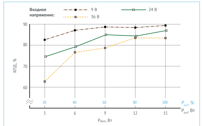
Рис. 16. КПД для VDRI15B24.
