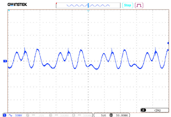
Рис. 47. Пульсации U_{\text{вых.ном}} . Масштаб 10 мВ/дел. Развертка 1 мкс/дел.
