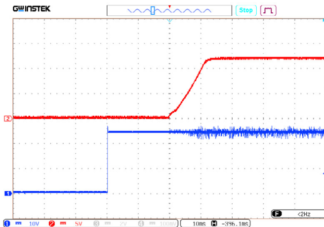
Рис. 50. Установление U_{\text{ВЫХ.НОМ}} с момента подачи U_{\text{ВХ.НОМ}} . Луч 1 (синий) – входное напряжение. Масштаб 10 В/дел. Луч 2 (красный) – выходное напряжение. Масштаб 5 В/дел. Развертка 10 мс/дел.
