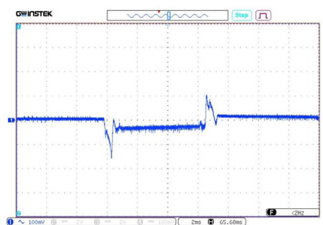
Рис. 41. Осциллограмма переходного отклонения выходного напряжения при скачкообразном изменении выходного тока с 50% до 100% и со 100% до 50%.
