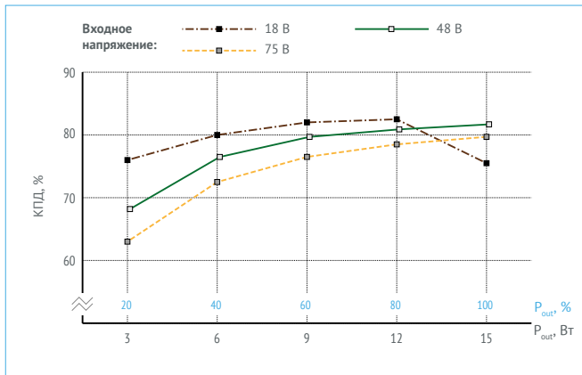
Рис. 18. КПД для VDRI15W3,3.
