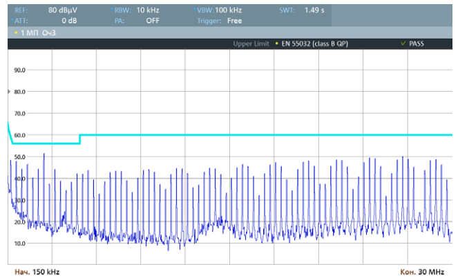
Рис. 57. Спектрограмма работы VDRI15B48 по схеме включения [Рис. 4], измерения произведены в соответствии с EN 55032 Class B (0,15–30 МГц).
