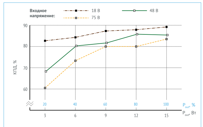
Рис. 23. КПД для VDRI15W24.
