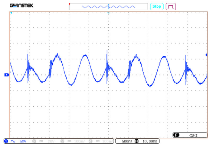
Рис. 55. Пульсации U_{\text{вых,ном}} . Масштаб 5 мВ/дел. Развертка 0,5 мкс/дел.
