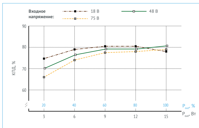
Рис. 11. КПД для VDRI15B33.
