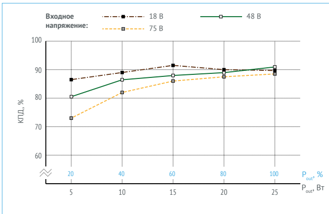
Рис. 35. КПД для VDRI25W15.
