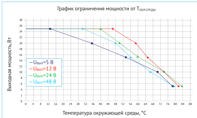
Рис. 38. График ограничения мощности от T_{окр.среды} без применения внешнего радиатора. Для модулей VDR125B с входной сетью «В», при U_{ВХ}=24 В .
