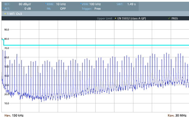
Рис. 56. Спектрограмма работы VDRI15B48 по схеме включения [Рис. 3], измерения произведены в соответствии с EN 55032 Class A (0,15–30 МГц).
