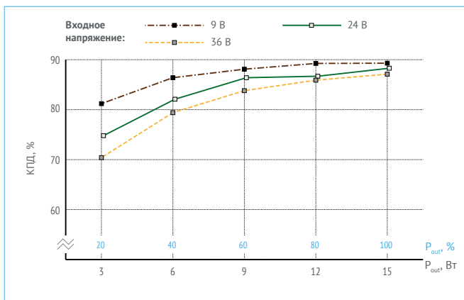
Рис. 14. КПД для VDRI15B12.
