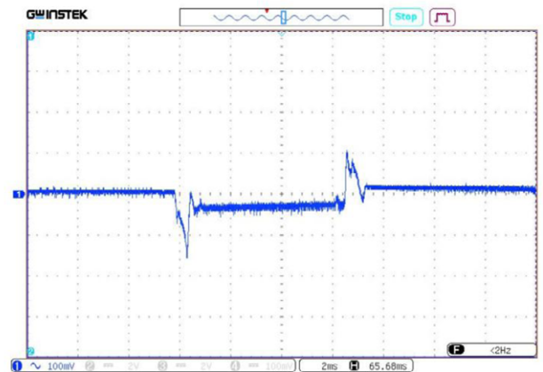
Рис. 45. Осциллограмма переходного отклонения выходного напряжения при скачкообразном изменении выходного тока с 50% до 100% и со 100% до 50%. Масштаб 100 мВ/дел. Развертка 2 мкс/дел.
