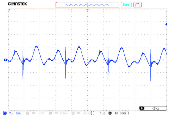
Рис. 43. Осциллограмма пульсаций U_{\text{вых.ном}} . Масштаб 5 мВ/дел. Развертка 1 мкс/дел.
