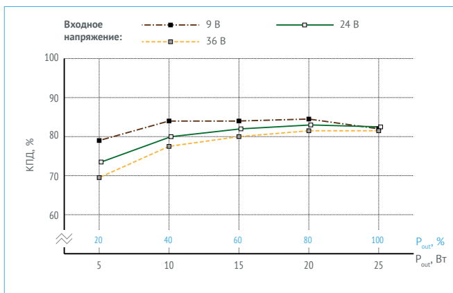
Рис. 25. КПД для VDRI25B3,3.
