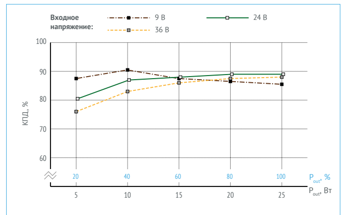
Рис. 28. КПД для VDRI25B15.
