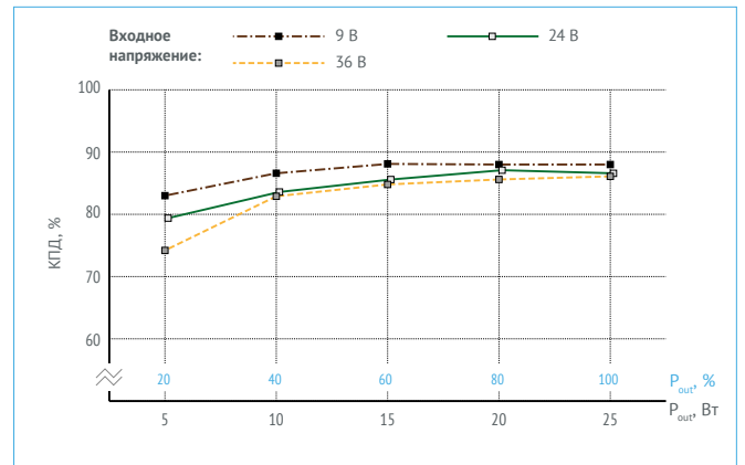
Рис. 30. КПД для VDRI25B48.
