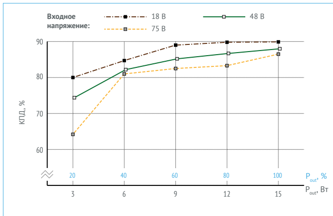
Рис. 24. КПД для VDRI15W48.
