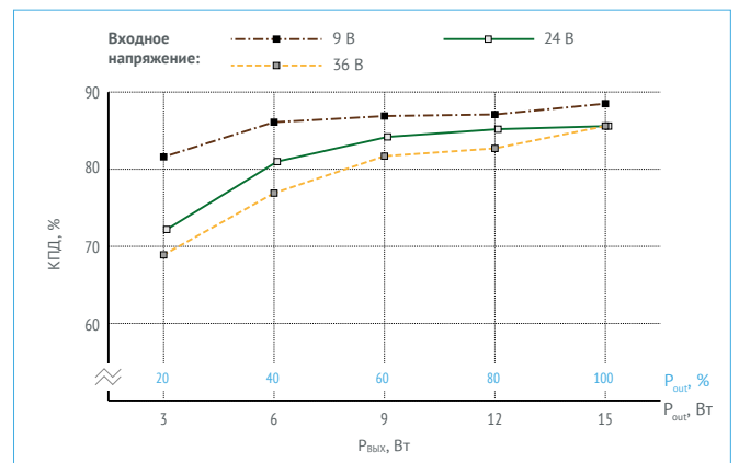
Рис. 17. КПД для VDRI15B48.
