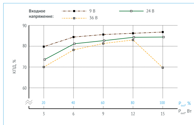
Рис. 12. КПД для VDRI15B05.
