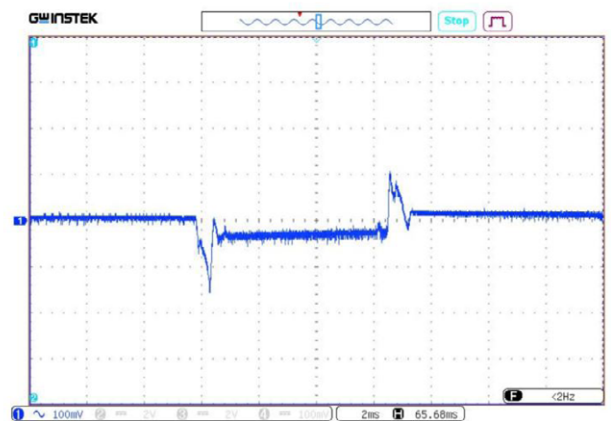
Рис. 49. Осциллограмма переходного отклонения выходного напряжения при скачкообразном изменении выходного тока с 50% до 100% и со 100% до 50%. Масштаб 100 мВ/дел. Развертка 2 мкс/дел.
