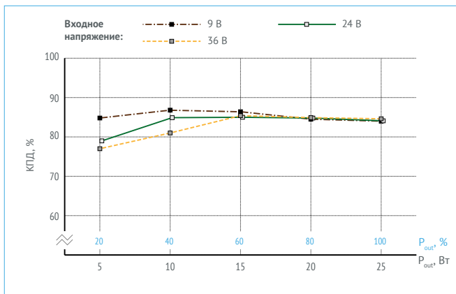
Рис. 26. КПД для VDRI25B05.
