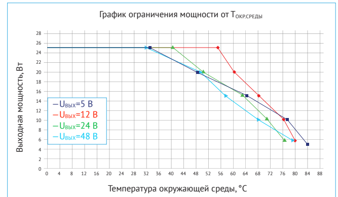
Рис. 39. График ограничения мощности от T_{окр.среды} без применения внешнего радиатора. Для модулей VDR125W с входной сетью «W», при U_{ВХ}=48 В .
