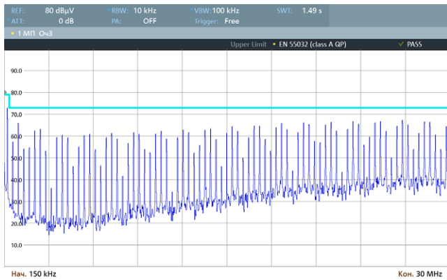
Рис. 62. Спектрограмма работы VDRI25W48 по схеме включения [Рис. 3], измерения произведены в соответствии с EN 55032 Class A (0,15–30 МГц).
