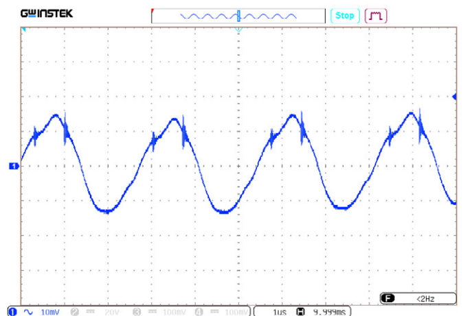
Рис. 51. Пульсации U_{\text{ВЫХ.НОМ}} . Масштаб 10 мВ/дел. Развертка 1 мкс/дел.
