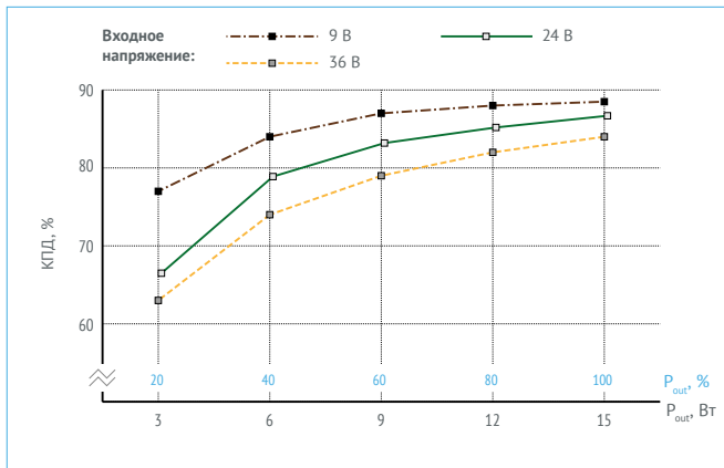
Рис. 13. КПД для VDRI15B09.
