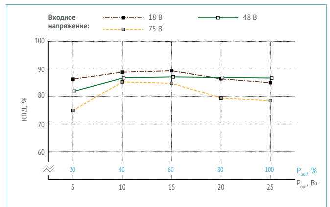
Рис. 32. КПД для VDRI25W05.
