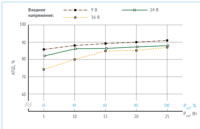
Рис. 29. КПД для VDRI25B24.
