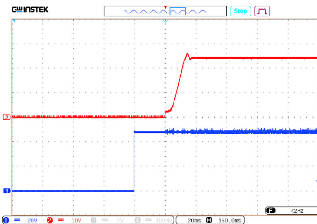
Рис. 46. Установление U_{\text{вых.ном}} с момента подачи U_{\text{вх.ном}} . Луч 1 (синий) – входное напряжение. Масштаб 20 В/дел. Луч 2 (красный) – выходное напряжение. Масштаб 10 В/дел. Развертка 20 мс/дел.
