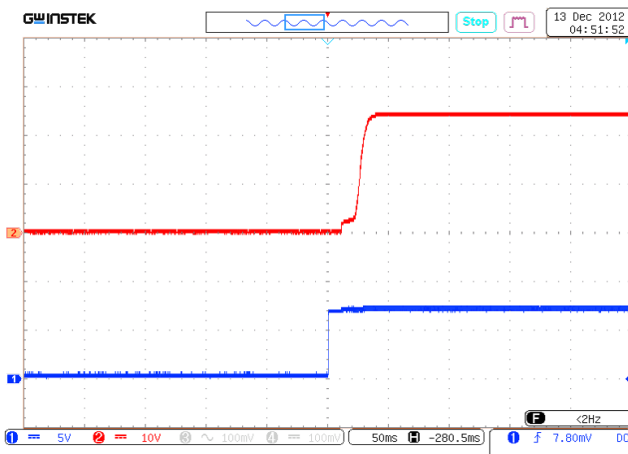
Рис. 32. Установление U_{\text{вых.ном}} с момента подачи сигнала ДУ (соединение выводов «ВКЛ» и «-ВХ».) Луч 1 (синий) – входное напряжение. Масштаб 5 В/дел. Луч 2 (красный) – выходное напряжение. Масштаб 10 В/дел. Развертка 50 мс/дел.
