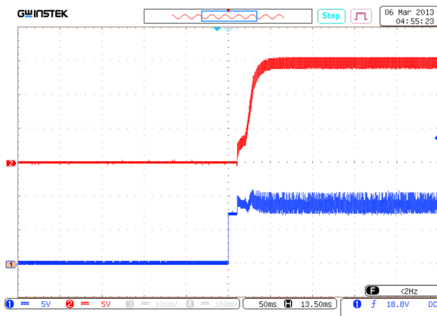
Рис. 24. Установление U_{ВЫХ.НОМ} с момента подачи сигнала ДУ (размыкание выводов «ДУ» и «ВХ»). Луч 1 (синий) — напряжение на выводе «ДУ». Масштаб 5 В/дел. Луч 2 (красный) — выходное напряжение. Масштаб 5 В/дел. Развертка 50 мс/дел.
