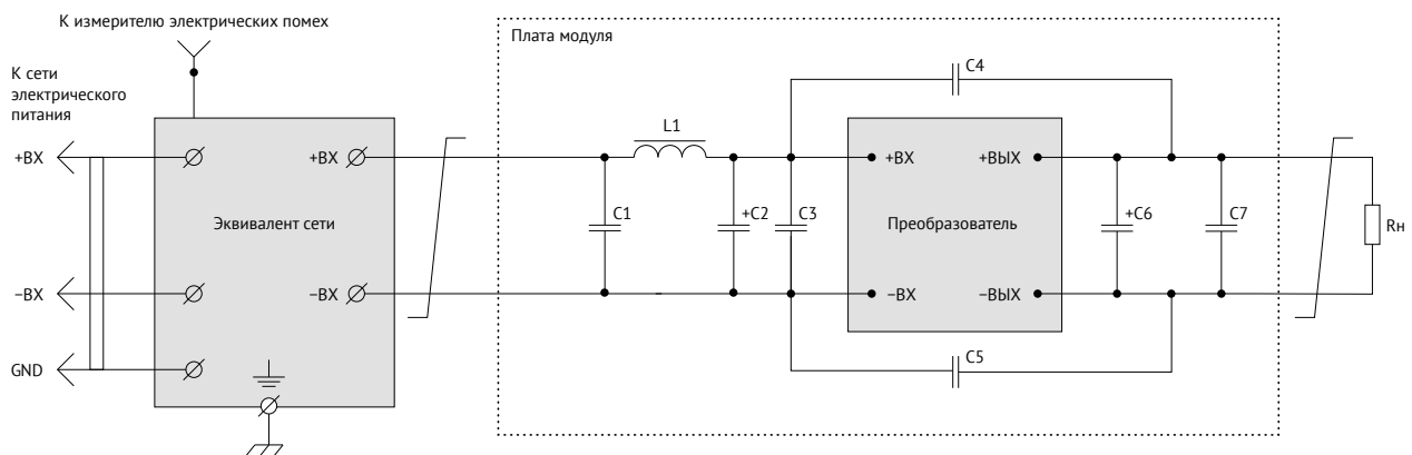
Рис. 3. Схема включения VDRI40, VDRI60 для соответствия стандарту EN 55032 Class A.
