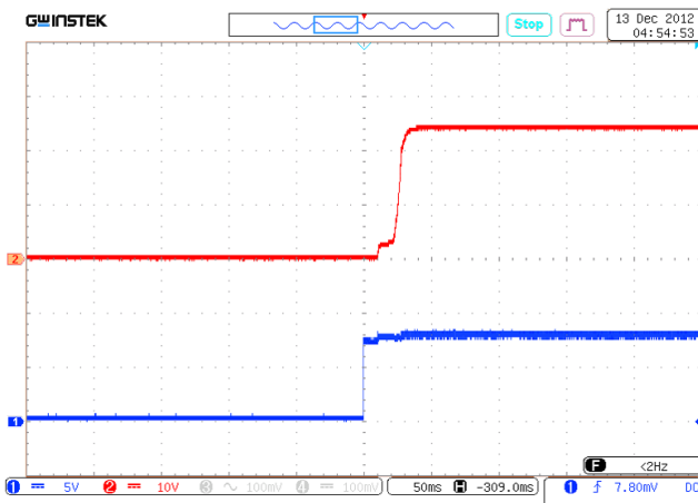
Рис. 36. Установление U_{\text{вых.ном}} с момента подачи сигнала ДУ (соединение выводов «ВКЛ» и «-ВХ».) Луч 1 (синий) – входное напряжение. Масштаб 5 В/дел. Луч 2 (красный) – выходное напряжение. Масштаб 10 В/дел. Развертка 50 мс/дел.
