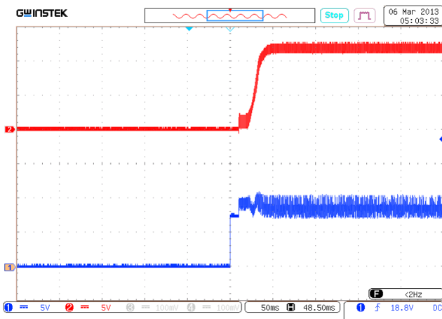
Рис. 28. Установление U_{ВЫХ.НОМ} с момента подачи сигнала ДУ (соединение выводов «ДУ» и «-ВХ».) Луч 1 (синий) – входное напряжение. Масштаб 5 В/дел. Луч 2 (красный) – выходное напряжение. Масштаб 5 В/дел. Развертка 50 мс/дел.
