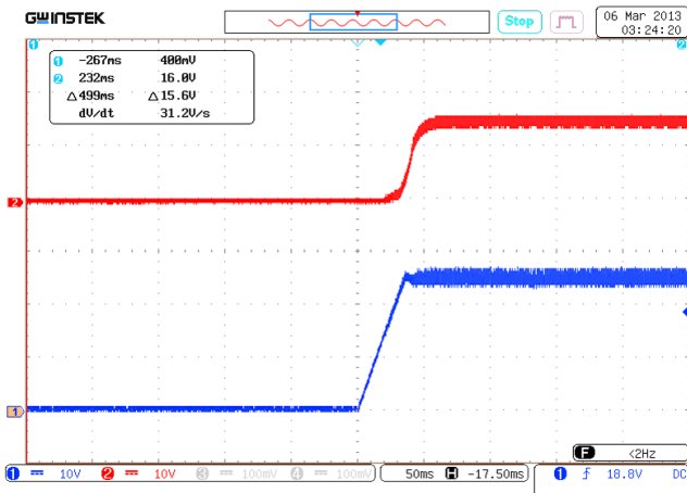
Рис. 26. Установление U_{ВЫХ.НОМ} с момента подачи U_{ВХ.НОМ} . Луч 1 (синий) – входное напряжение. Масштаб 10 В/дел. Луч 2 (красный) – выходное напряжение. Масштаб 10 В/дел. Развертка 50 мс/дел.
