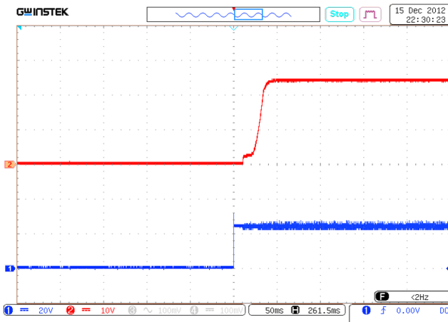
Рис. 34. Установление U_{\text{вых.ном}} с момента подачи U_{\text{вх.ном}} . Луч 1 (синий) – входное напряжение. Масштаб 20 В/дел. Луч 2 (красный) – выходное напряжение. Масштаб 10 В/дел. Развертка 50 мс/дел.
