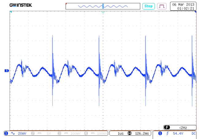
Рис. 27. Осциллограмма пульсаций U_{ВЫХ.НОМ} . Масштаб 20 мВ/дел. Развертка 1 мкс/дел.
