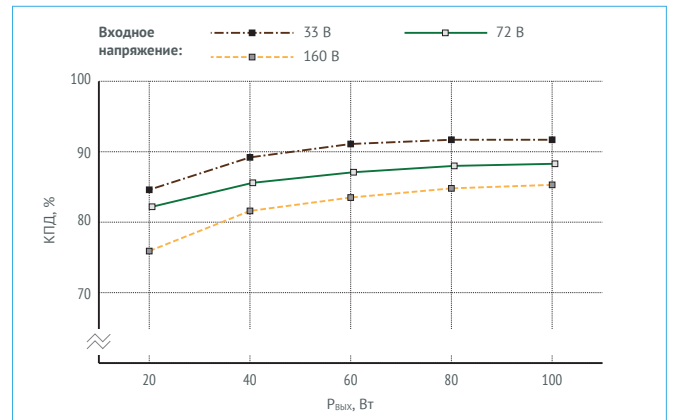
Рис. 20. КПД для VDRW100N24.
