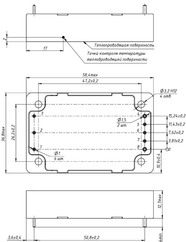
Рис. 30. Исполнение 1/4 Brick.
