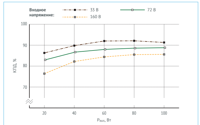
Рис. 19. КПД для VDRW100N15.
