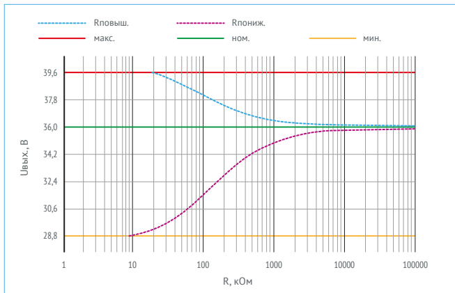
Рис. 13. График зависимости для VDRW50N36.
