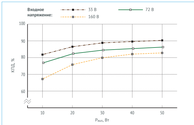
Рис. 17. КПД для VDRW50N05.
