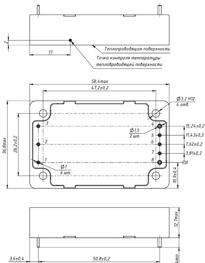
Рис. 30. Исполнение 1/4 Brick.
