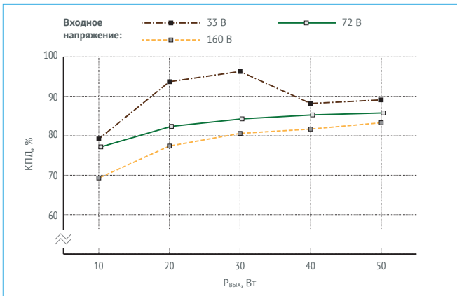
Рис. 21. КПД для VDRW50N36.
