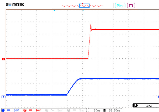
Рис. 26. Установление U_{\text{вых.ном}} с момента подачи U_{\text{вх.ном}} .
