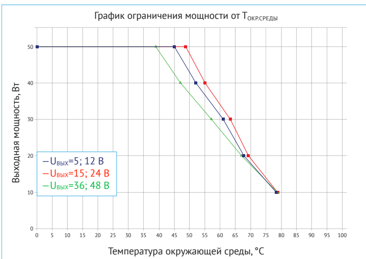
Рис. 23. График ограничения мощности от T_{окр.среды} без применения внешнего радиатора. Для модулей VDRW50N с входной сетью «N», при U_{вх}=72 В .
