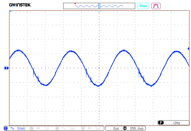
Рис. 27. Пульсации U_{\text{вых.ном}} .
