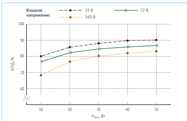
Рис. 18. КПД для VDRW50N12.
