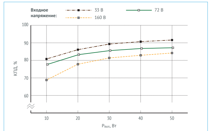
Рис. 19. КПД для VDRW50N15.
