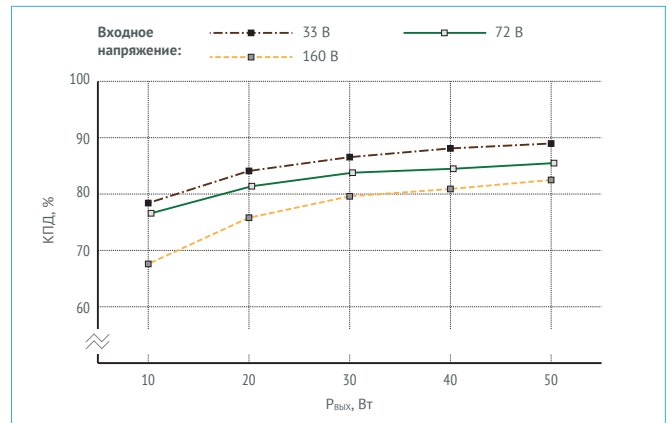
Рис. 22. КПД для VDRW50N48.
