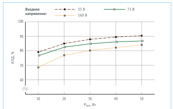
Рис. 20. КПД для VDRW50N24.
