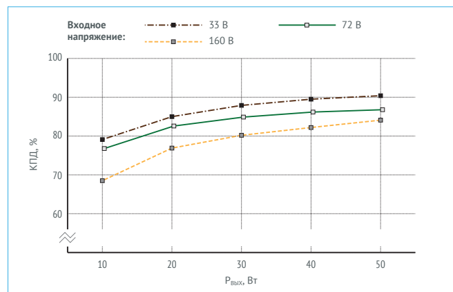
Рис. 20. КПД для VDRW50N24.
