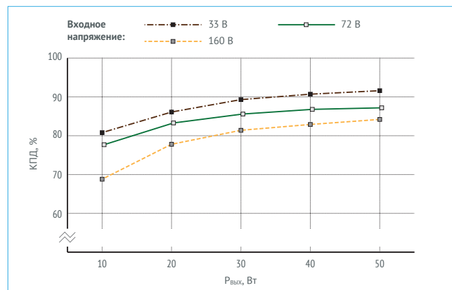
Рис. 19. КПД для VDRW50N15.
