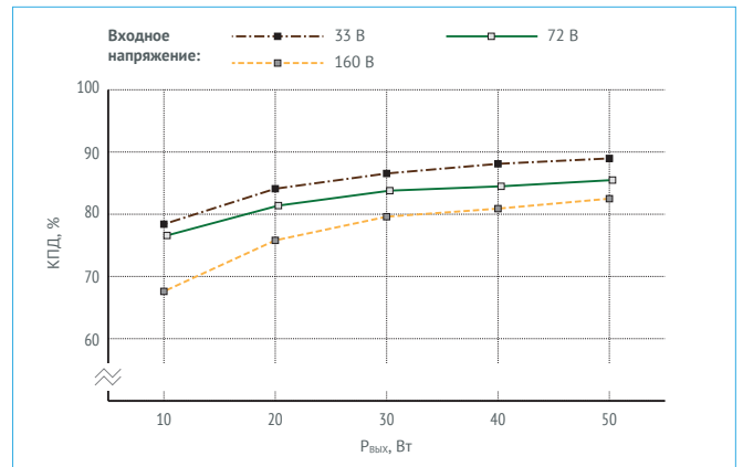
Рис. 22. КПД для VDRW50N48.
