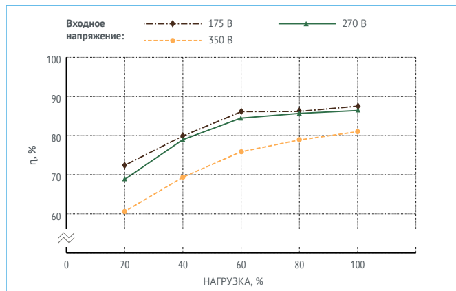
Рис. 5. КПД VDV(HV)40-1M28.
