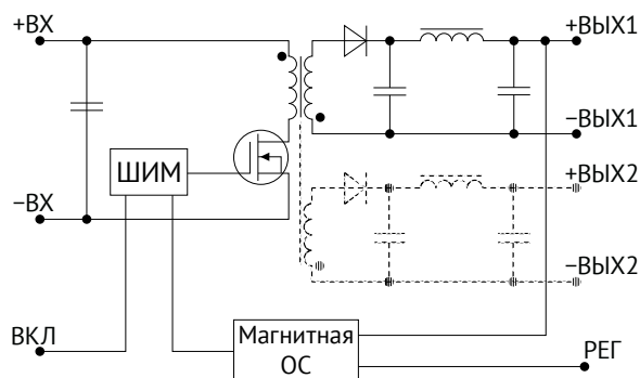
Рис. 1. Топология VDV(HV)40.
