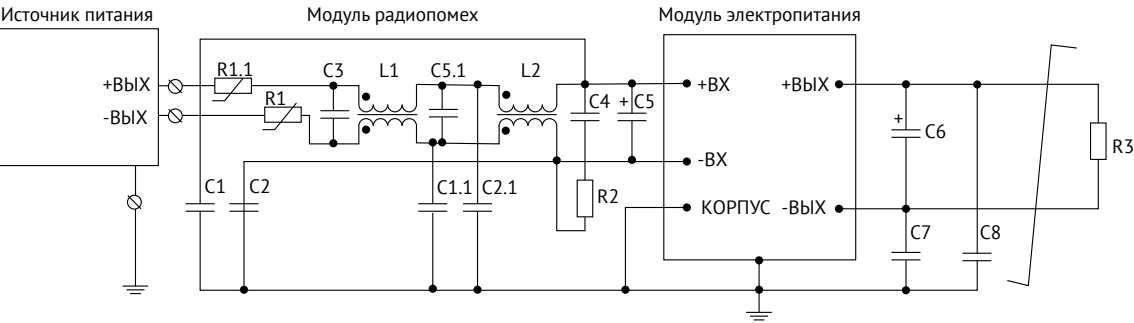
Рис. 2. Типовая схема подключения для одноканального модуля.
