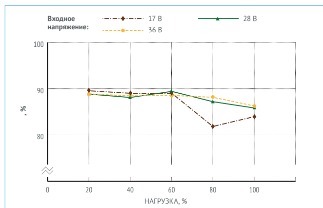
Рис. 7. КПД VDV1000-1V28.
