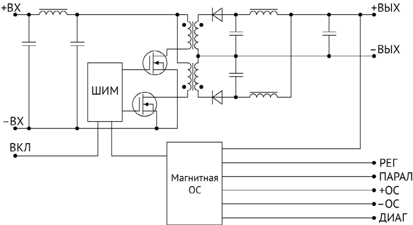
Рис. 1. Топология VDV1000.
