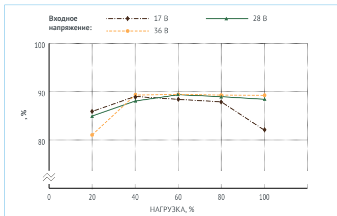
Рис. 7. КПД VDV160-1V28.
