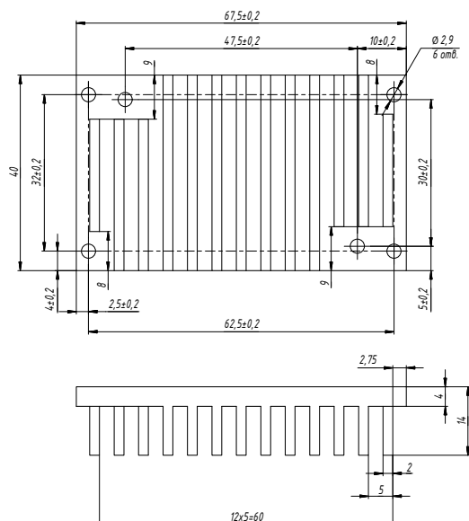
Рис. 10 (а). ТУЛВ. 752695.004.
