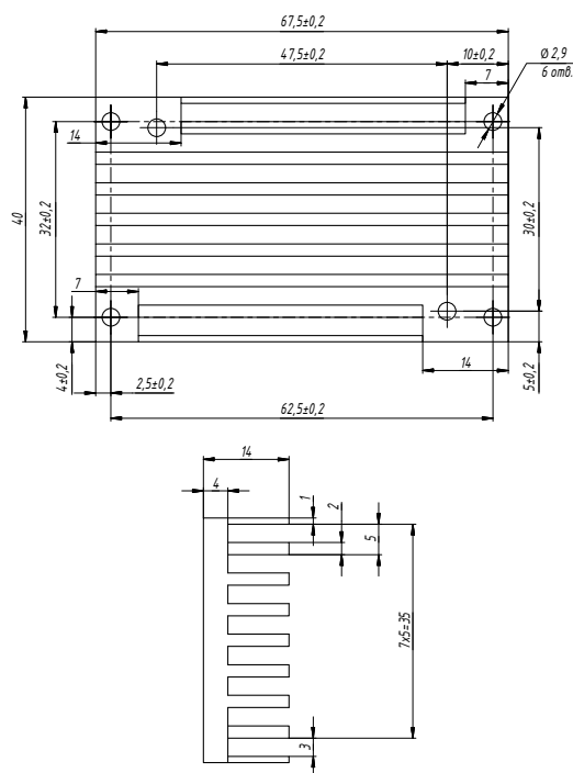
Рис. 10 (в). ТУЛВ. 752695.005.
