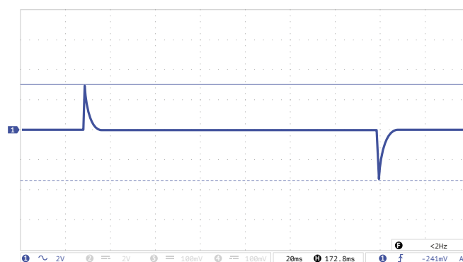
Рис. 7 (г). Осциллограмма переходного отклонения выходного напряжения при изменении выходного тока.
