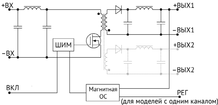
Рис. 1. Топология VDV50.
