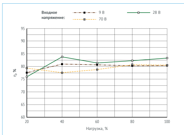
Рис. 6. КПД VDV-1E12.
