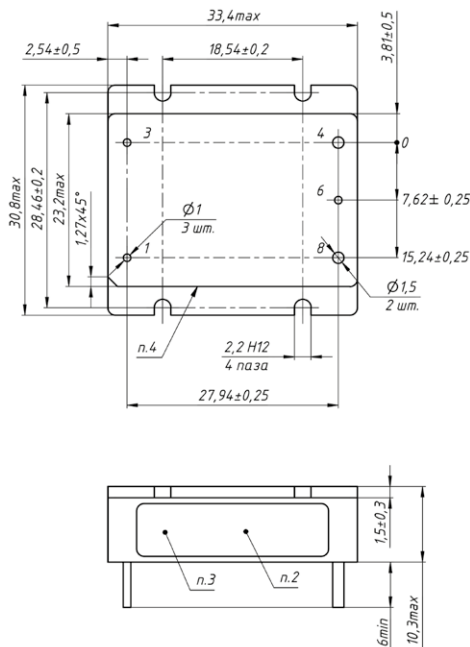
Рис. 3. Исполнение VFD07.
